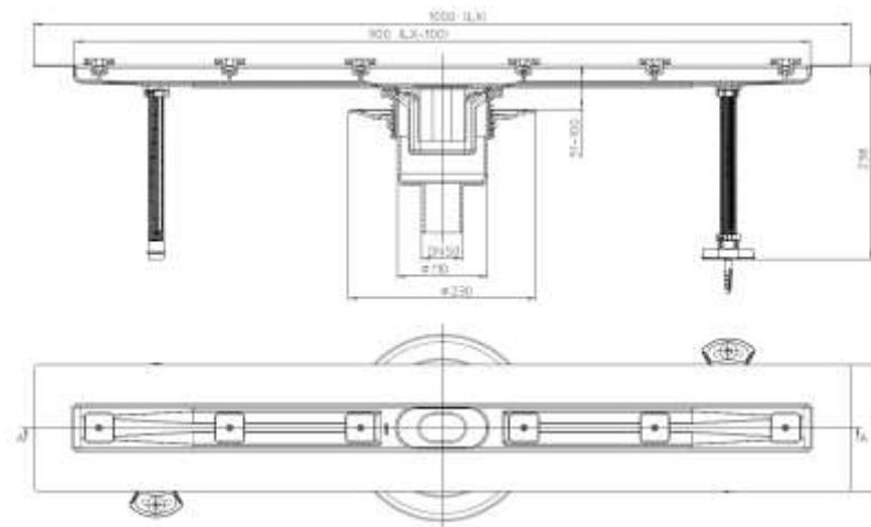
Рис. 1. Корпус лотка HL50FV.0/100.
